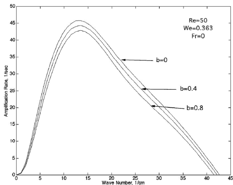
Figura 2.2.3: Efeito da velocidade de regressão da superfície do bloco de combustível sólido na taxa de amplificação das instabilizações ( b é o parâmetro de velocidade de regressão da superfície do bloco de combustível sólido) (retirado de Karabeyoglu; Cantwell [4])
