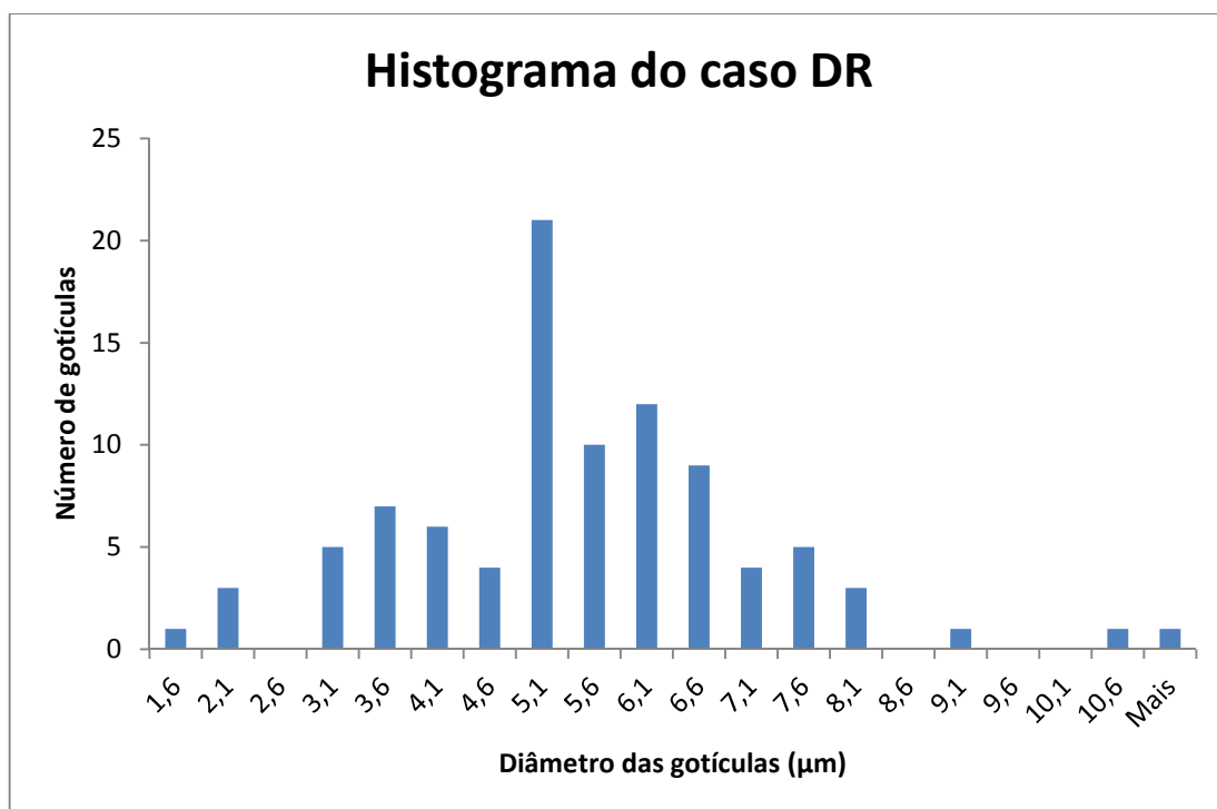
Figura B.15: Histograma dos diâmetros das gotículas do caso DR
