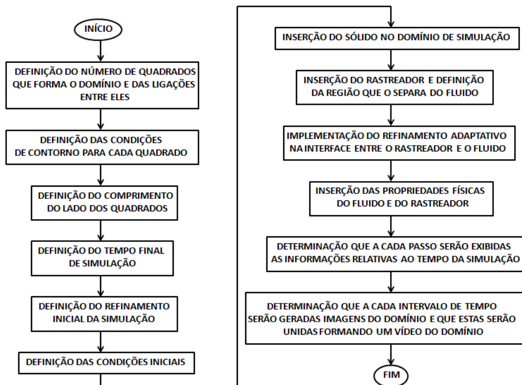
Figura 3.1.1: Descrição da sequência lógica utilizada no desenvolvimento do código para simular o fenômeno de entrainment com o programa Gerris Flow Solver
