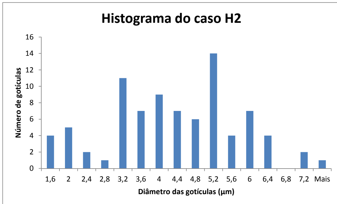
Figura B.7: Histograma dos diâmetros das gotículas do caso H2
