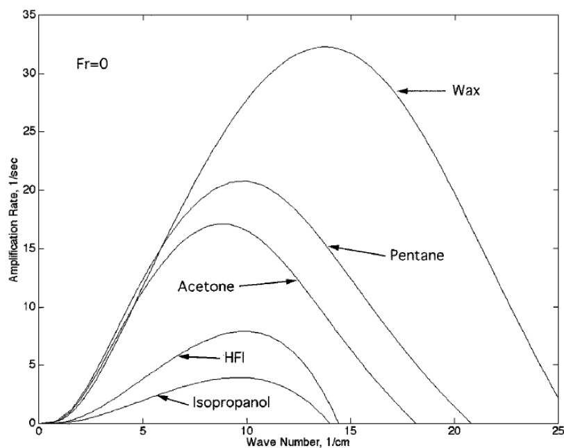
Figura 2.2.4: Efeito do combustível sólido na taxa de amplificação das instabilizações (retirado de Karabeyoglu; Cantwell [4])
