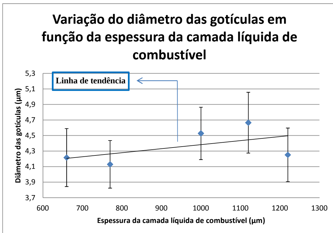
Figura 4.4.1: Representação gráfica dos diâmetros médios e dos intervalos de confiança dos casos utilizados na análise do efeito da espessura da camada líquida de combustível
