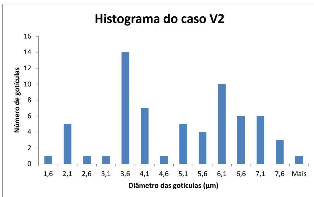
Figura B.3: Histograma dos diâmetros das gotículas do caso V2
