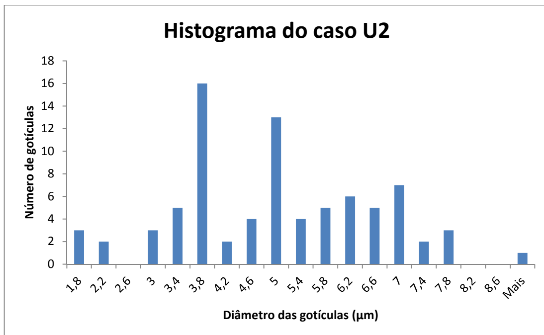
Figura B.11: Histograma dos diâmetros das gotículas do caso U2
