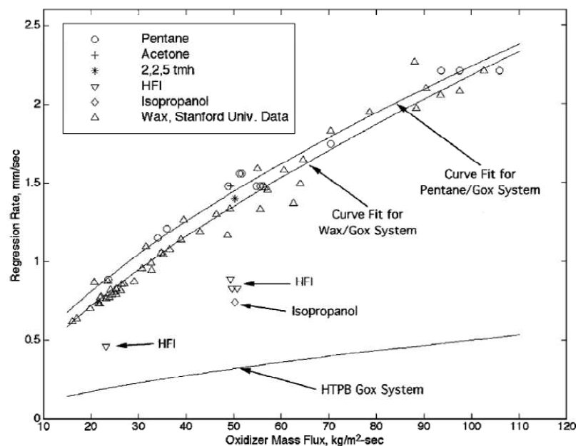
Figura 2.1.1: Velocidades de regressão da superfície do bloco de combustível sólido obtidas para vários combustíveis sólidos (retirado de Karabeyoglu; Altman; Cantwell [3])
