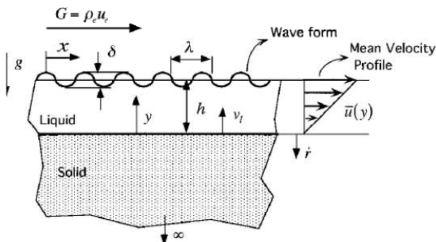
Figura 2.2.1: Modelo de estabilidade estudado (retirado de Karabeyoglu; Cantwell [4])
