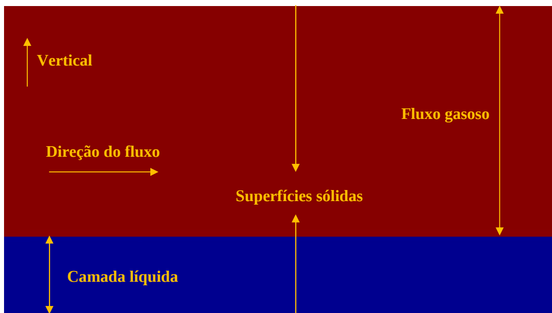
Figura 3.1.2.1: Geometria criada para representar bidimensionalmente a câmara de combustão de um motor híbrido (obtido com Gerris Flow Solver [6])
