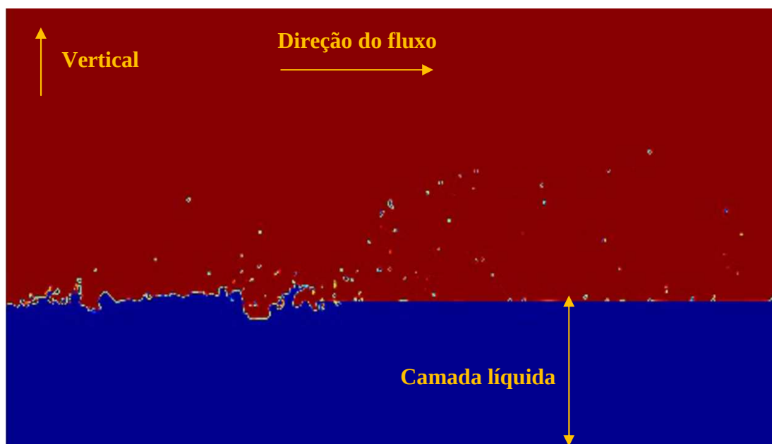
Figura 3.1.7.2: Aumento da área destacada da figura 3.1.7.1 (obtido com Gerris Flow Solver [6])
