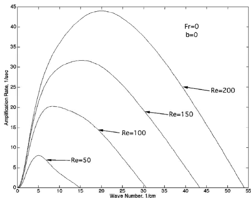
Figura 2.2.2: Efeito do número de Reynolds do fluxo gasoso na taxa de amplificação das instabilizações (retirado de Karabeyoglu; Cantwell [4])
