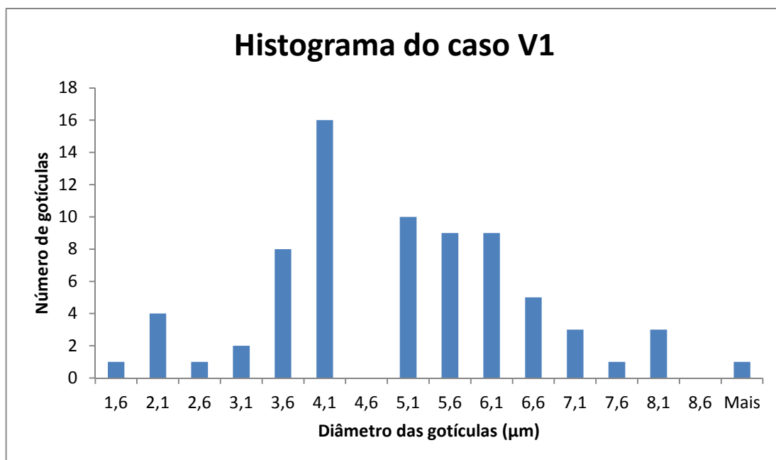
Figura B.2: Histograma dos diâmetros das gotículas do caso V1
