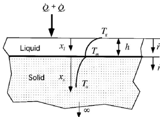
Figura 2.1.2: Modelo térmico utilizado para o desenvolvimento da expressão da espessura da camada líquida (retirado de Karabeyoglu; Altman; Cantwell [3])
