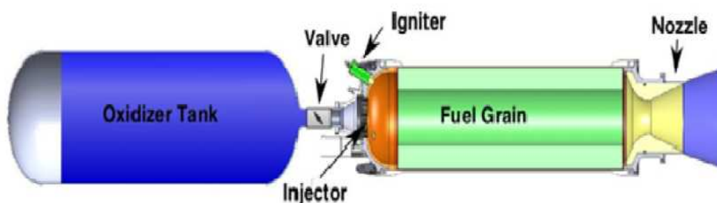
Figura 1.1.1.1: Configuração clássica de um motor a propulsão híbrida
