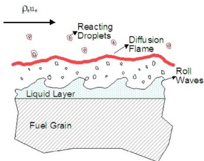
Figura 1.1.2.1: Ilustração do fenômeno de entrainment (retirado de Franchi [2])
