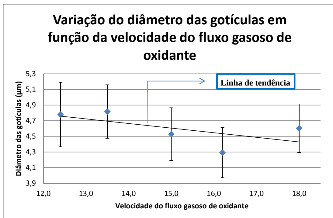
Figura 4.5.1: Representação gráfica dos diâmetros médios e dos intervalos de confiança dos casos utilizados na análise do efeito da velocidade do fluxo gasoso de oxidante
