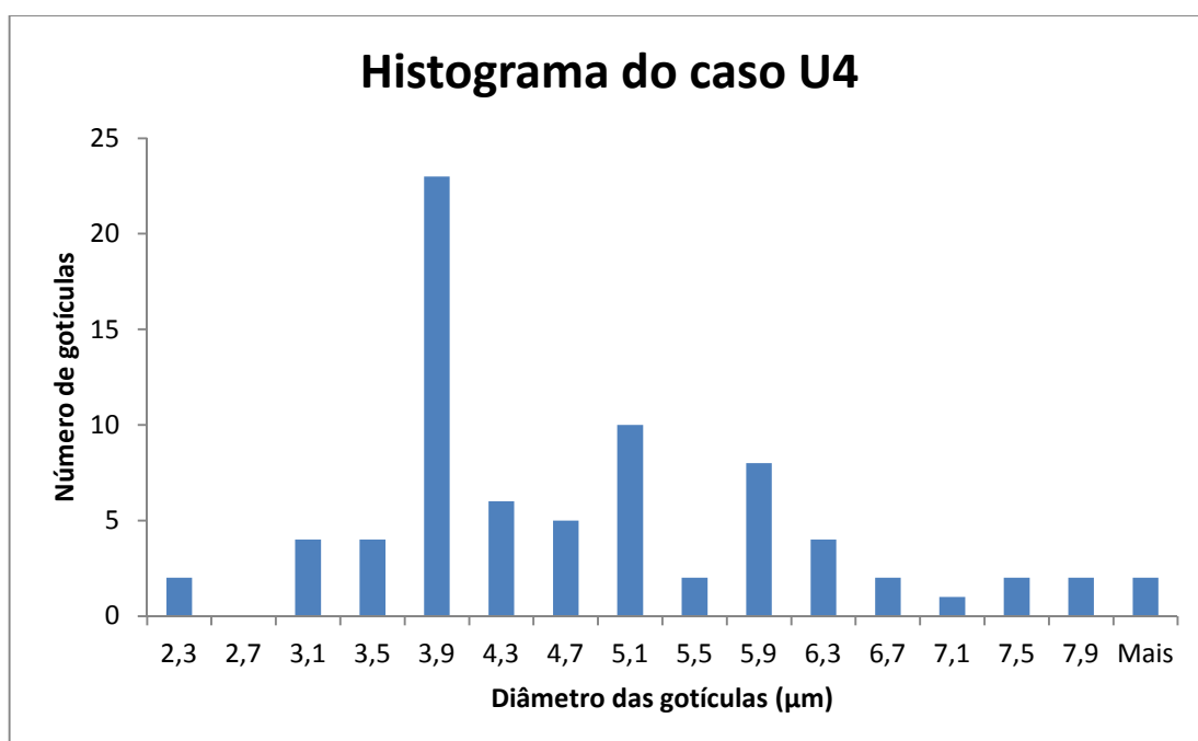
Figura B.13: Histograma dos diâmetros das gotículas do caso U4
