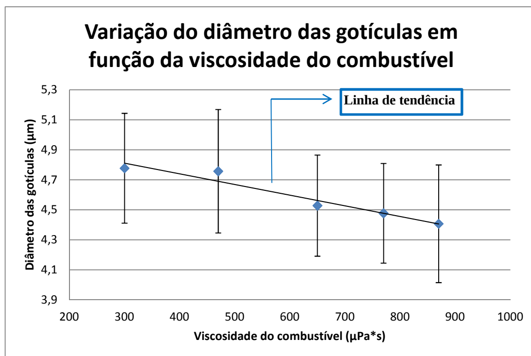
Figura 4.3.1: Representação gráfica dos diâmetros médios e dos intervalos de confiança dos casos utilizados na análise do efeito da viscosidade do combustível
