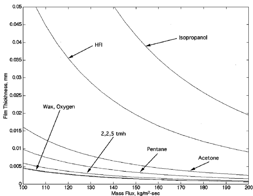
Figura 2.1.3: Condições críticas para a ocorrência do fenômeno de entrainment para cada combustível sólido (retirado de Karabeyoglu; Altman; Cantwell [3])
