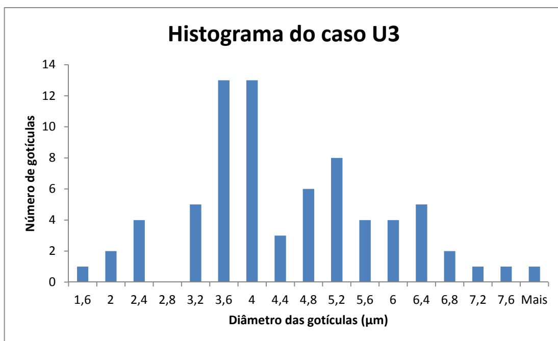
Figura B.12: Histograma dos diâmetros das gotículas do caso U3
