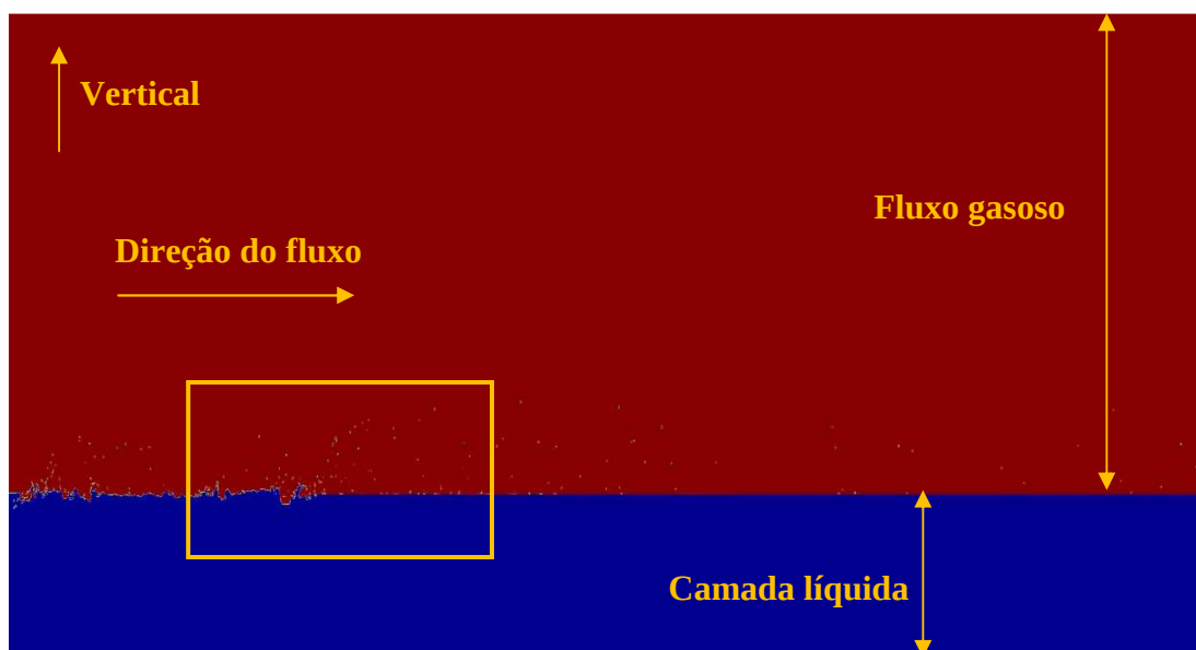
Figura 3.1.7.1: Ilustração do fenômeno de entrainment obtido com a simulação do código desenvolvido para o programa Gerris Flow Solver (obtido com Gerris Flow Solver [6])
