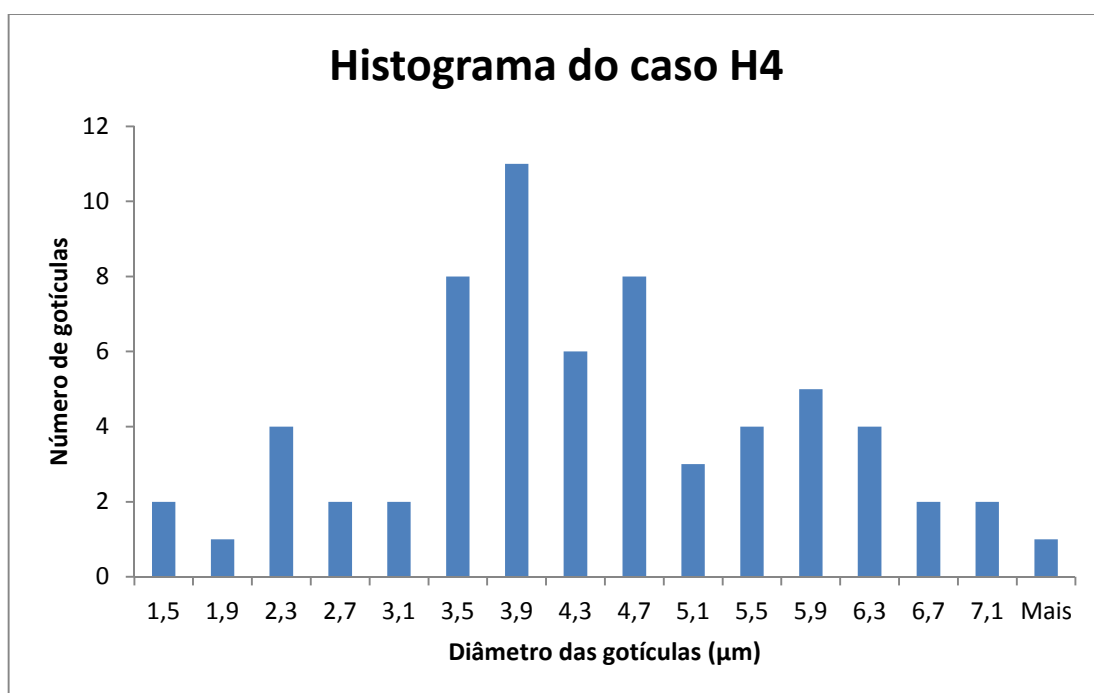
Figura B.9: Histograma dos diâmetros das gotículas do caso H4
