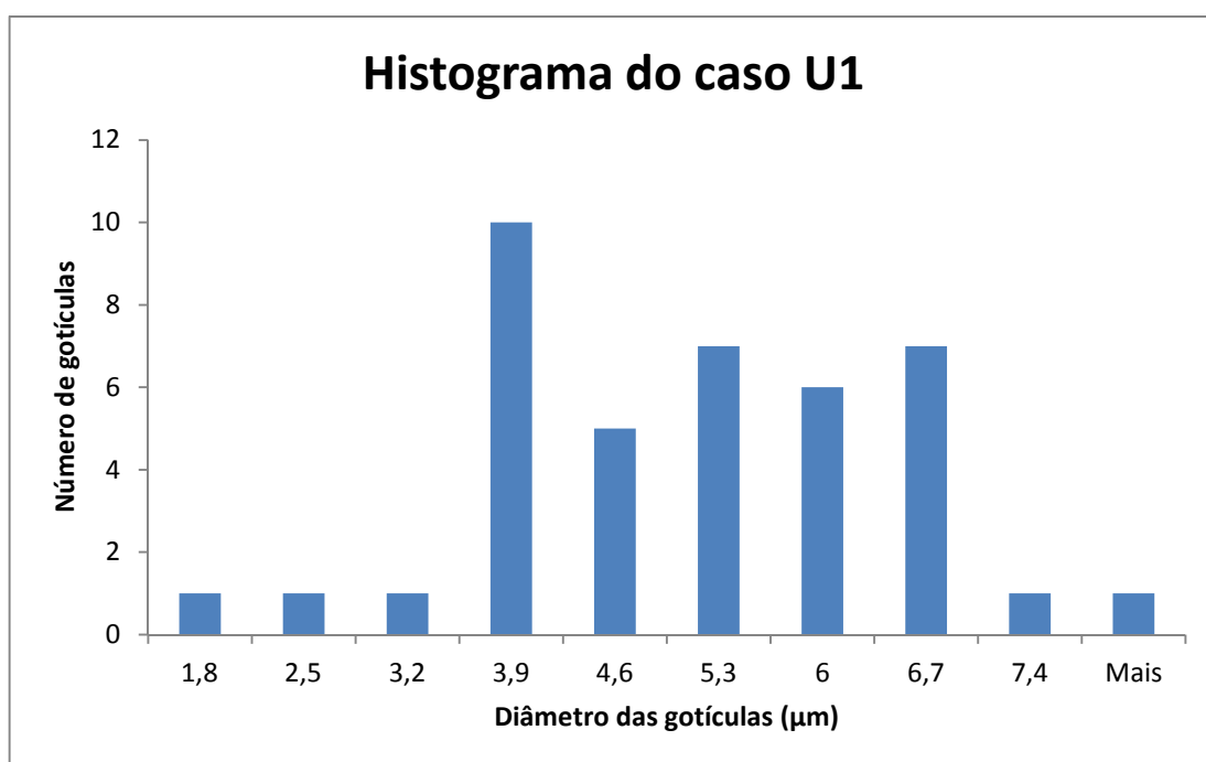
Figura B.10: Histograma dos diâmetros das gotículas do caso U1
