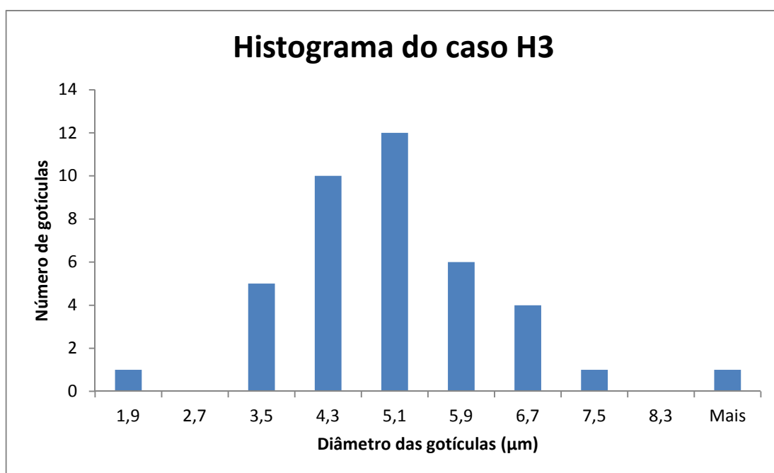
Figura B.8: Histograma dos diâmetros das gotículas do caso H3
